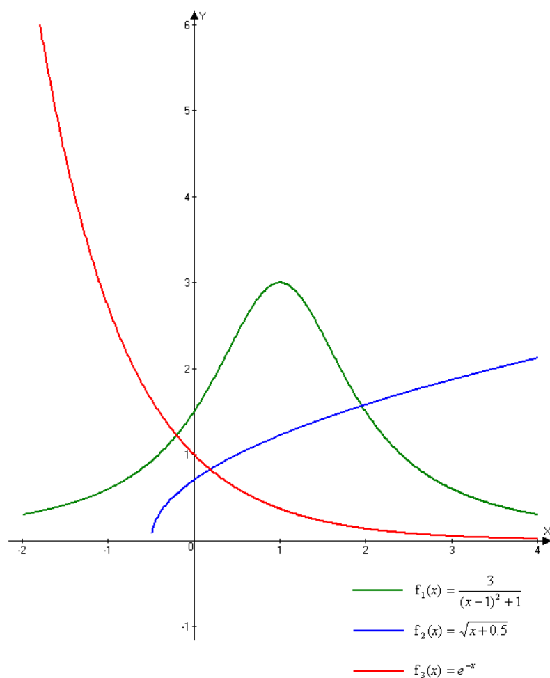
Рис. 1 – Плоская фигура, ограниченная графиками заданных уравнений.
