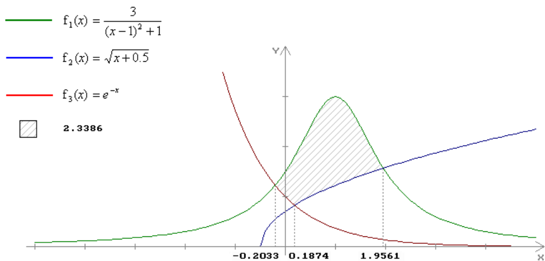
Рис. 2 – Абсциссы точек пересечения графиков, полученные в результате численных расчетов.
